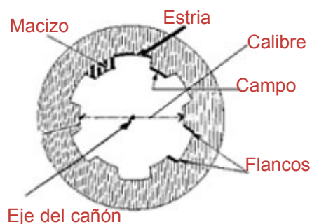
FIGURA 6.2. Partes del estriado de un cañón y representación del calibre.
