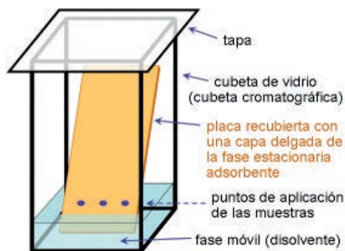
FIGURA 2.4. Cromatografía en capa fina.
