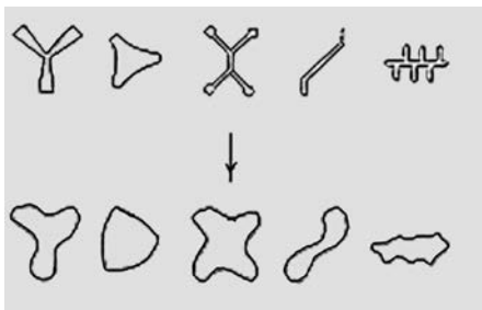
FIGURA 4.3. Parte superior, formas de hilera de fibras manufacturadas. Parte inferior, secciones transversales sin orificios (izquierda) y con orificios (derecha).
