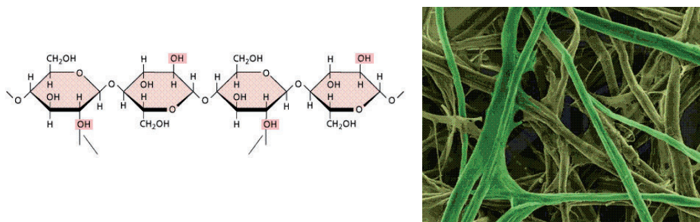
FIGURA 3.8. Polímero de celulosa unidades de glucosa (A) y fibras de celulosa en el papel (B).
