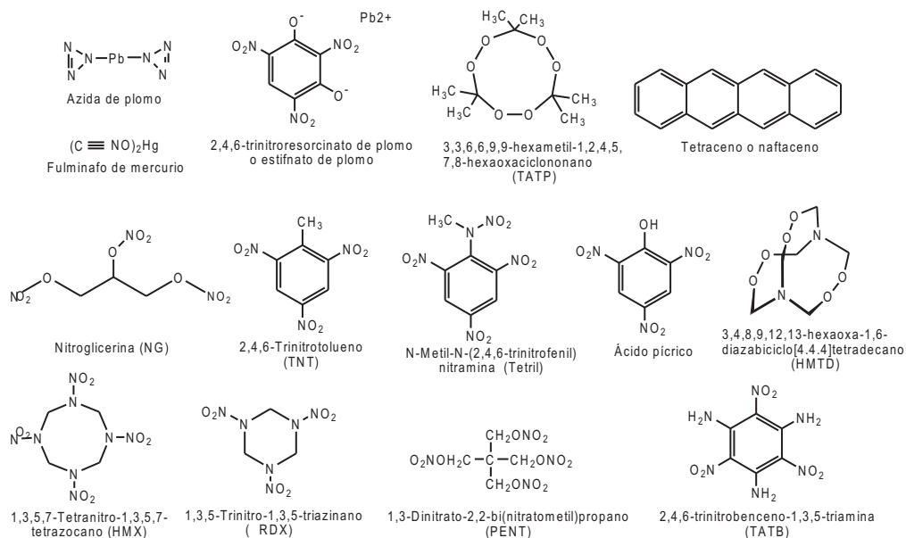
FIGURA 5.6. Estructura molecular de diferentes explosivos.
