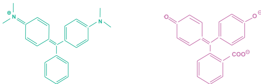
FIGURA 8.2. Estructura del verde de malaquita y de la fenolftaleína (formas iónicas).
