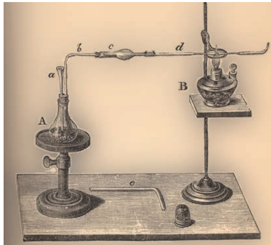
FIGURA 10.5. Aparato ideado por Marsh para realizar el test de arsénico.
