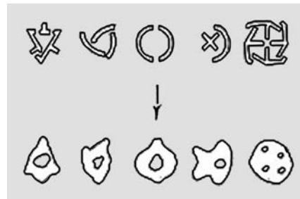
FIGURA 4.3. Parte superior, formas de hilera de fibras manufacturadas. Parte inferior, secciones transversales sin orificios (izquierda) y con orificios (derecha).
