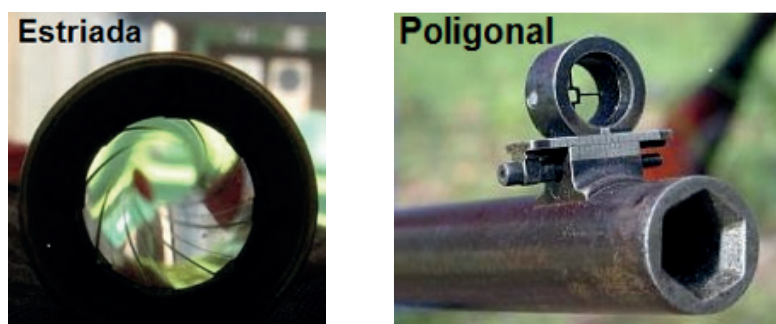
FIGURA 6.1. Diferentes tipos de ánimas.
