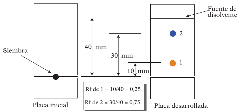
FIGURA 4.13. Determinación experimental del R_f .
