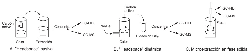
FIGURA 5.4. Técnicas de "Headspace" (A y B) y microextracción en fase sólida, C.
