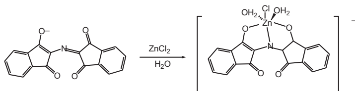
FIGURA 7.12. Formación del complejo de zinc de color naranja, por reacción entre el cloruro de cinc y la ninhidrina (color violeta/azul).
