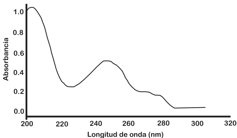
FIGURA 2.9. Espectro UV de la estricnina.
