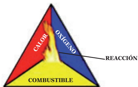
FIGURA 5.1. Triángulo del fuego.
