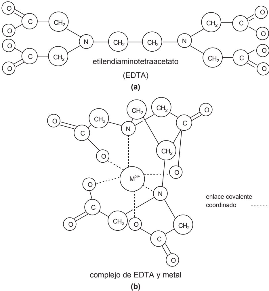
FIGURA 10.2. (a) Molécula de EDTA - (b) Molécula de EDTA envolviendo un ion metálico, M^{3+} , estableciendo con él 6 enlaces covalentes coordinados (líneas de puntos), formando un quelato.
