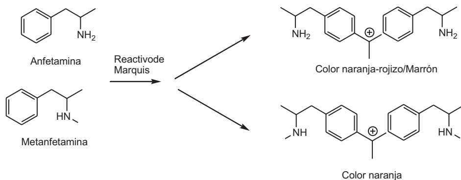
FIGURA 9.10. Mecanismo de reacción propuesto para la Anfetamina y la Metanfetamina con el reactivo de Marquis.
