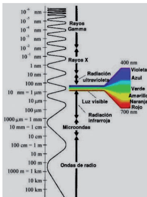
FIGURA 2.8. Espectro de las radiaciones electromagnéticas.
