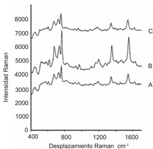
FIGURA 3.6. Espectros Raman de tres tintas distintas, A, B y C.
