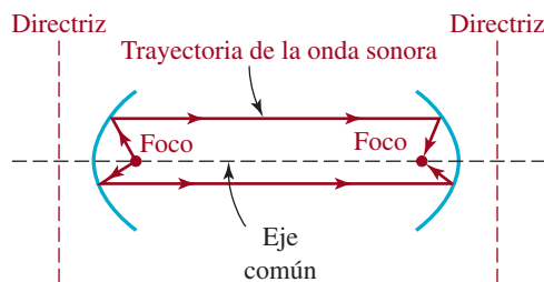
FIGURA 11.1.15 Superficies reflectoras parabólicas del problema 59
