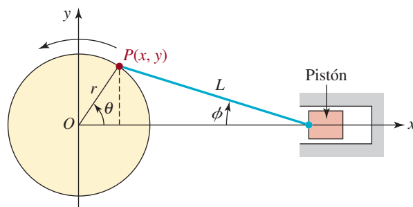
FIGURA 11.5.11 Mecanismo de cigüeñal del problema 35
