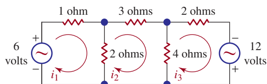
FIGURA 13.1.6 Circuito para el problema 40
