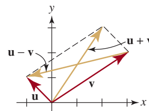
FIGURA 12.4.10 Suma y diferencia de vectores del ejemplo 3
