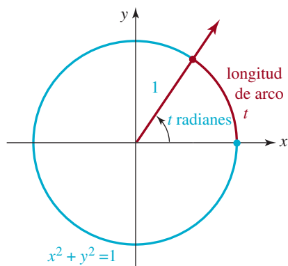
FIGURA 9.1.1 Círculo unitario
