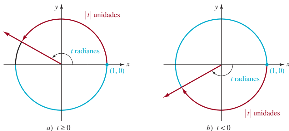
FIGURA 9.1.2 El ángulo de t radianes subtiende un arco de longitud |t| unidades
