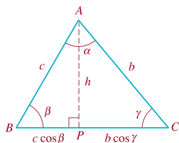
FIGURA 10.4.2 Triángulo acutángulo
