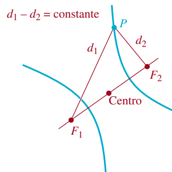
FIGURA 11.3.1 Una hipérbola
