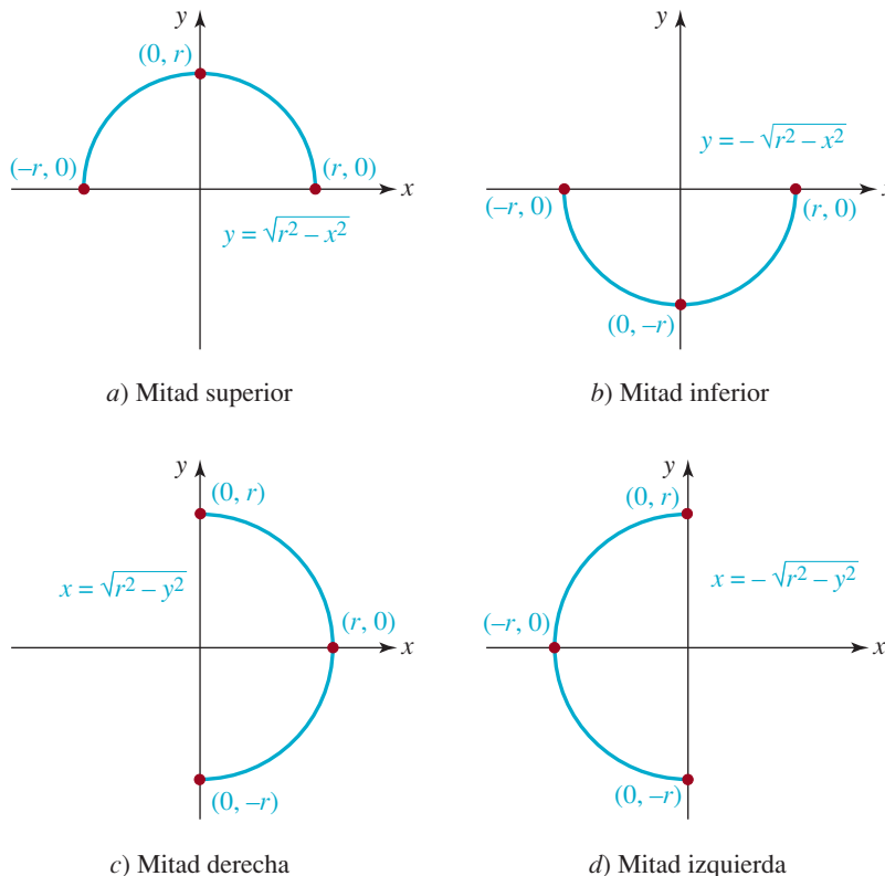
FIGURA 4.2.6 Semicírculos
