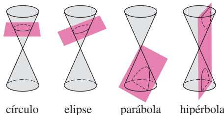
FIGURA 11.1.1 Secciones cónicas
