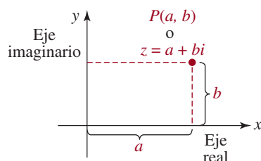
FIGURA 10.6.1 Plano complejo
