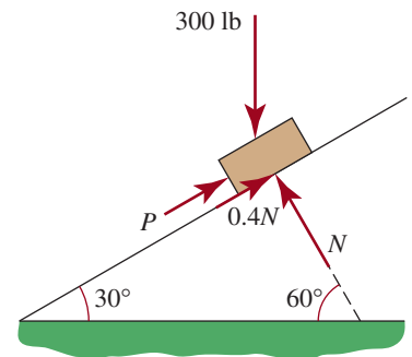
FIGURA 13.1.3 Plano inclinado para el ejemplo 5
