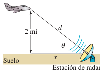
FIGURA 10.2.6 Avión del ejemplo 5
