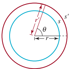
FIGURA 8.1.7 Círculos concéntricos
