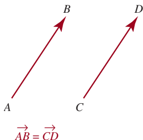
FIGURA 12.4.2 Vectores iguales
