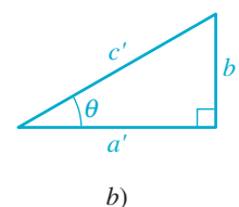
FIGURA 8.2.2 Triángulos semejantes
