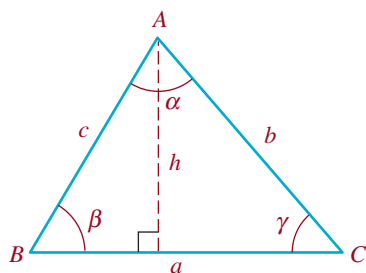
FIGURA 10.3.2 Triángulo agudo
