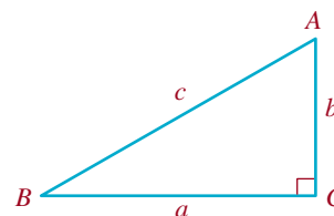
FIGURA 10.4.1 Triángulo rectángulo
