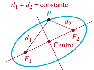
FIGURA 11.2.1 Una elipse
