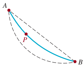
FIGURA 11.5.7 Cuenta deslizante
