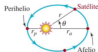
FIGURA 12.3.8 Órbita del satélite alrededor del Sol.
