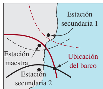
FIGURA 11.3.8 Concepto del LORAN
