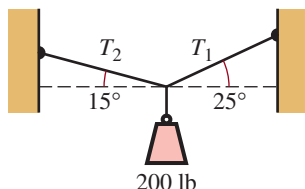
FIGURA 13.1.4 Cables para el problema 31
