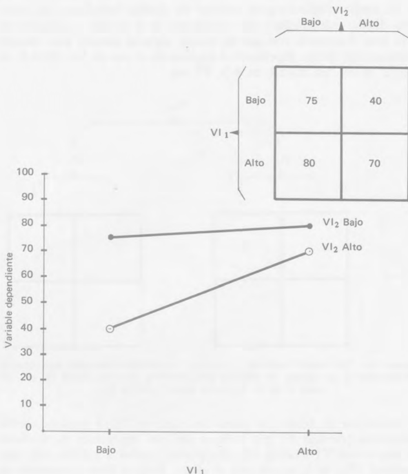
Figura 28. Datos ficticios que muestran el efecto de la interacción de las VI 1 y VI 2 sobre la VD. Los puntos representan las medias aritméticas de las condiciones.
