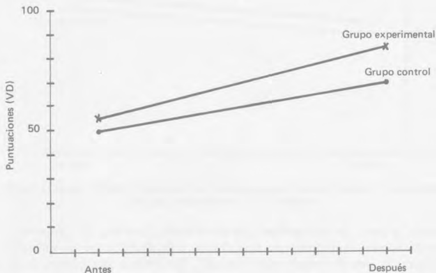
Figura 1. Datos ficticios que muestran un mayor aumento en el grupo experimental que en el grupo control.
