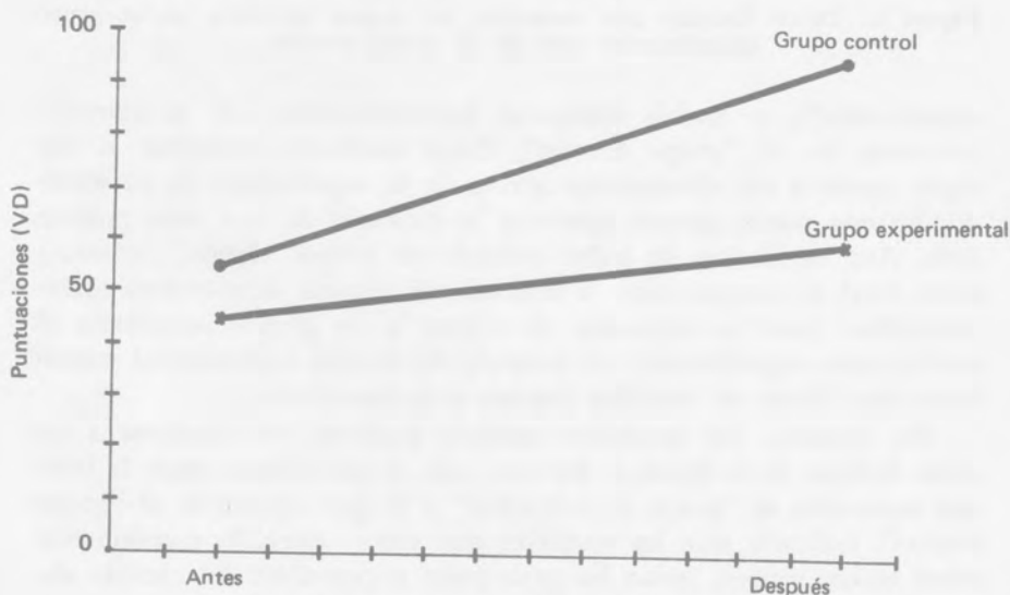
Figura 3. Datos ficticios que muestran un mayor aumento en el grupo control que en el grupo experimental.
