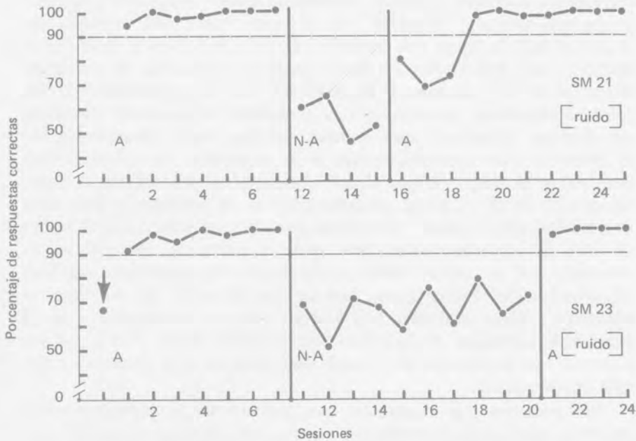
Figura 19. Adquisición del control de estímulos sobre las respuestas de unos monos, obtenida con las bocinas en la posición adyacente (A), y efectos de un cambio posadquisición a la posición no adyacente (N-A) seguidos por un regreso a la posición adyacente (A). Se usó reforzamiento no diferencial durante las tres fases del diseño. Los estímulos fueron ruido o tronidos de 10-khz (indicados para los animales individuales entre paréntesis). El punto marcado con una flecha (en SM 23) representa la conducta antes de la inclusión de los estímulos de sonidos. (Tomado de Downey y Harrison, Journal of the Experimental Analysis of Behavior , vol. 18, núm. 3, 1972, págs. 453-463. Copyright por la Society for the Experimental Analysis of Behavior, Inc.)
