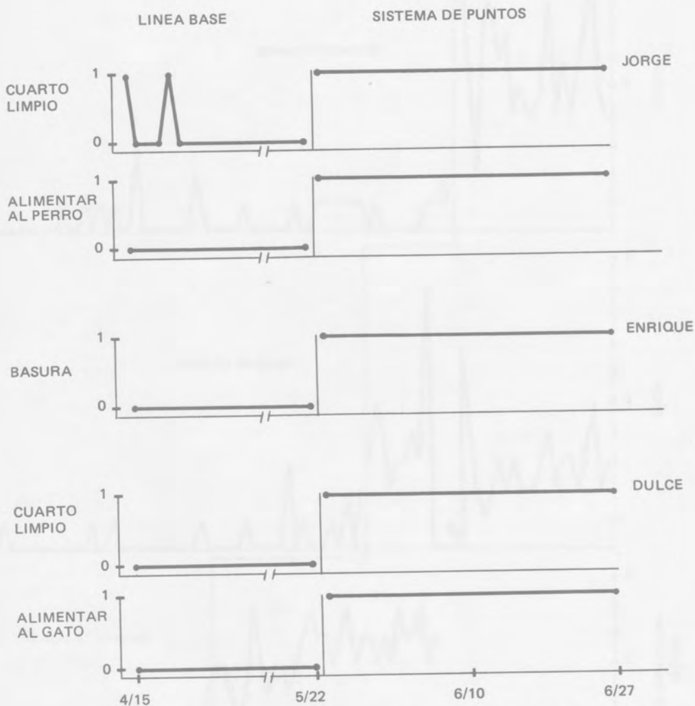
Figura 9. Efectos de la inclusión de un sistema de puntos para el mantenimiento de las conductas de tres niños (de 9, 5 y 8 años de edad), simultáneamente. (Tomado y adaptado de Christophersen, Arnold, Hill y Quillitch, Journal of Applied Behavior Analysis , vol. 5, núm. 4, verano de 1972, págs. 485-497. Copyright 1972 por la Society for the Experimental Analysis of Behavior, Inc.)
