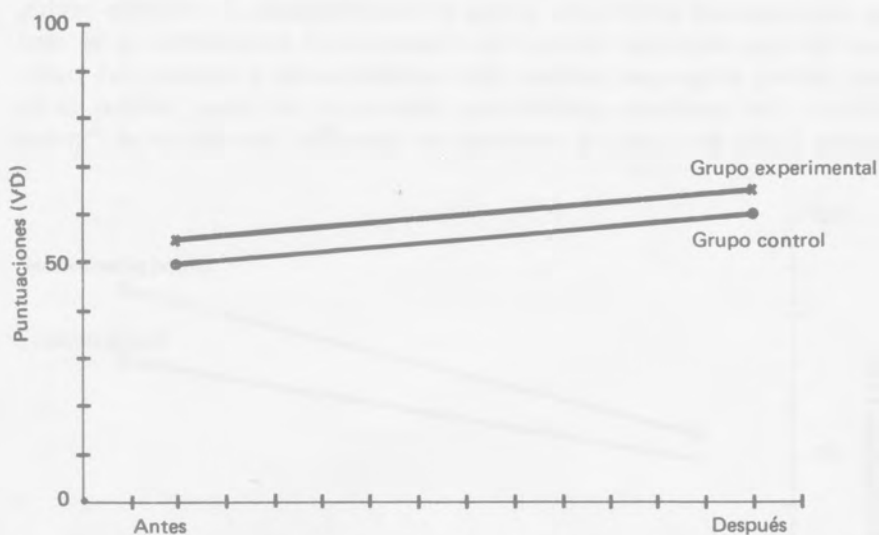
Figura 2. Datos ficticios que muestran un aumento similar entre el grupo control y el grupo experimental.
