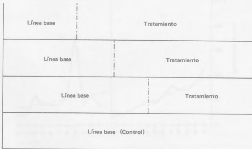
Figura 42. Diagrama del diseño experimental mixto
