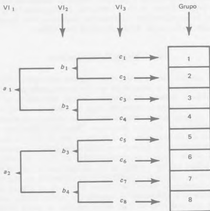
Figura 33. Esquema de un diseño jerárquico con tres VI: la primera con dos niveles, la segunda con cuatro niveles y anidada a la primera, y la tercera con ocho niveles y anidada a la segunda.
