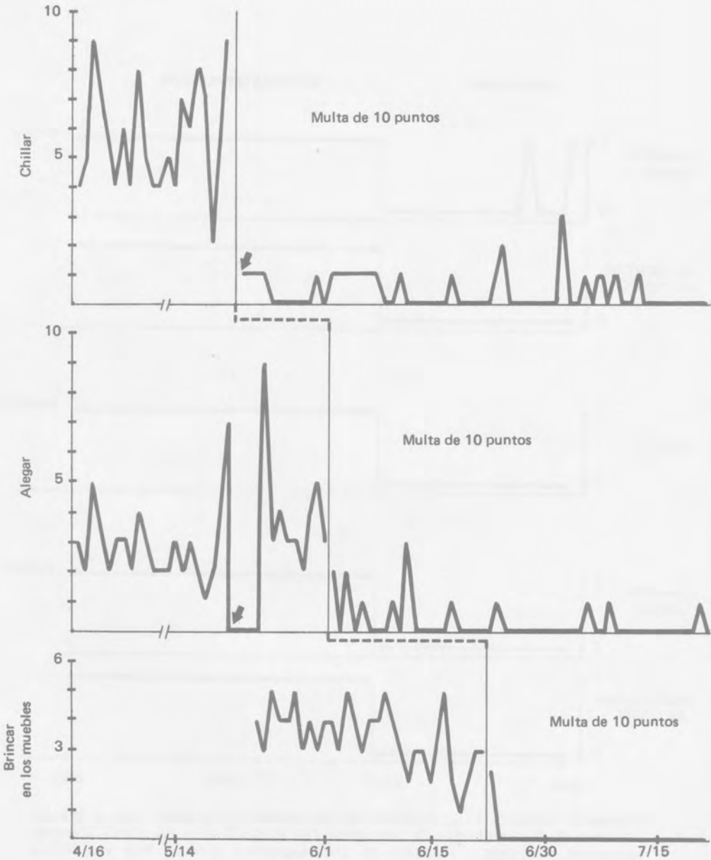
Fig. 10. Análisis de línea base múltiple de los efectos de la inclusión de multas de puntos sobre las conductas sociales de una niña de 8 años de edad. Las flechas indican cuándo se estableció el sistema de puntos para el mantenimiento de las conductas. (Tomado y adaptado de Christophersen, Arnold, Hill y Quilitch, Journal of Applied Behavior Analysis , vol. 5, núm. 4, invierno de 1972, págs. 485-497. Copyright 1972 por la Society for the Experimental Analysis of Behavior, Inc.)
