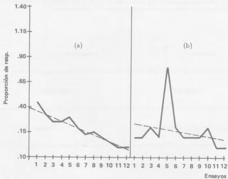
Figura 40 (a). Curva de posición serial obtenida con la serie completa de observaciones (40 observaciones) (b). Curva de posición serial obtenida exclusivamente con el bloque de observaciones más estables (10 observaciones).
