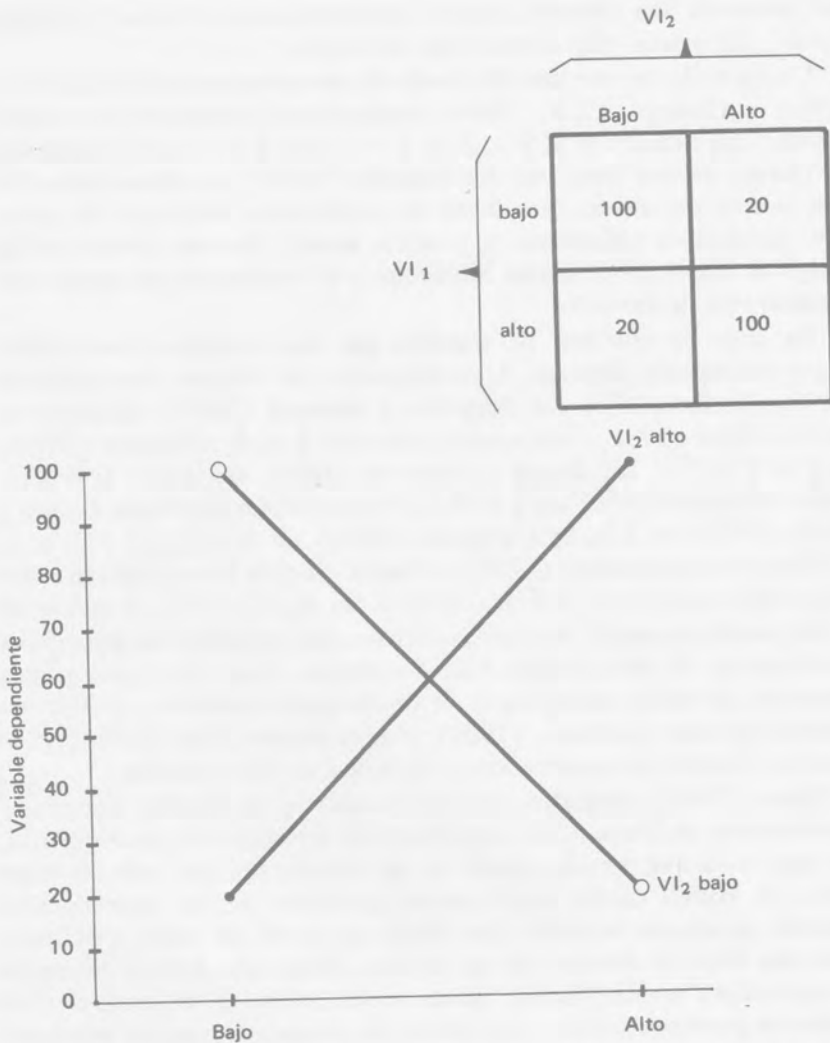
Figura 30. Datos ficticios y gráfica de un diseño factorial de 2 \times 2 que muestran una interacción extrema.
