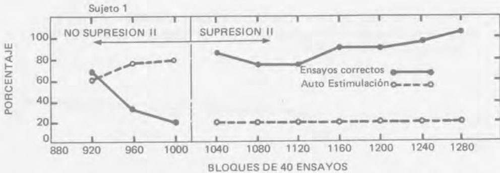
Figura 6. Porcentaje de ocurrencias de autoestimulación y de ensayos correctos para el sujeto 1 durante la segunda condición de "no supresión". A este sujeto se le aplicó una segunda condición de "supresión" de la autoestimulación. (Tomada y adaptada de Koegel y Covert, Journal of Applied Behavior Analysis , vol. 5, núm. 4, verano de 1972, págs. 381-387. Copyright 1972 de la Society for the Experimental Analysis of Behavior, Inc.)
