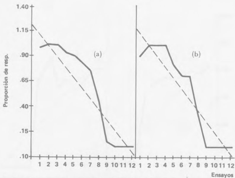
Figura 39 (a). Curva de posición serial obtenida de la serie completa de observaciones (40 observaciones) (b). Curva de posición serial obtenida exclusivamente con el bloque de observaciones más estables (10 observaciones)
