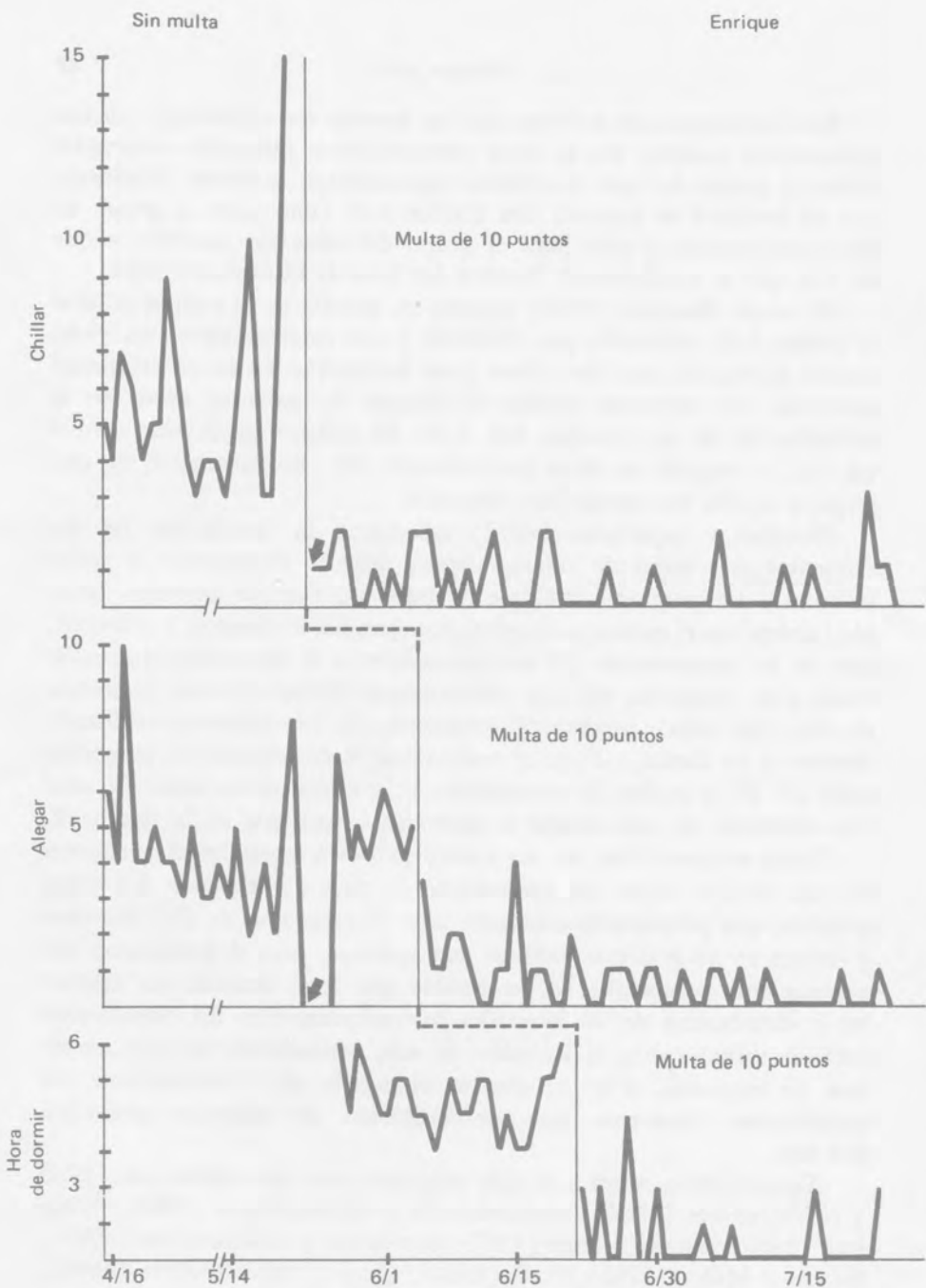
Figura 11. Análisis de línea base múltiple de los efectos de la inclusión de multas de puntos sobre las conductas sociales de un niño de 5 años de edad. Las flechas indican cuándo se estableció el sistema de puntos para el mantenimiento de las conductas. (Tomado y adaptado de Christophersen, Arnold, Hill y Quilitch, Journal of Applied Behavior Analysis , vol. 5, núm. 4, verano de 1972, págs. 485-497. Copyright 1972 por la Society for the Experimental Analysis of Behavior, Inc.)
