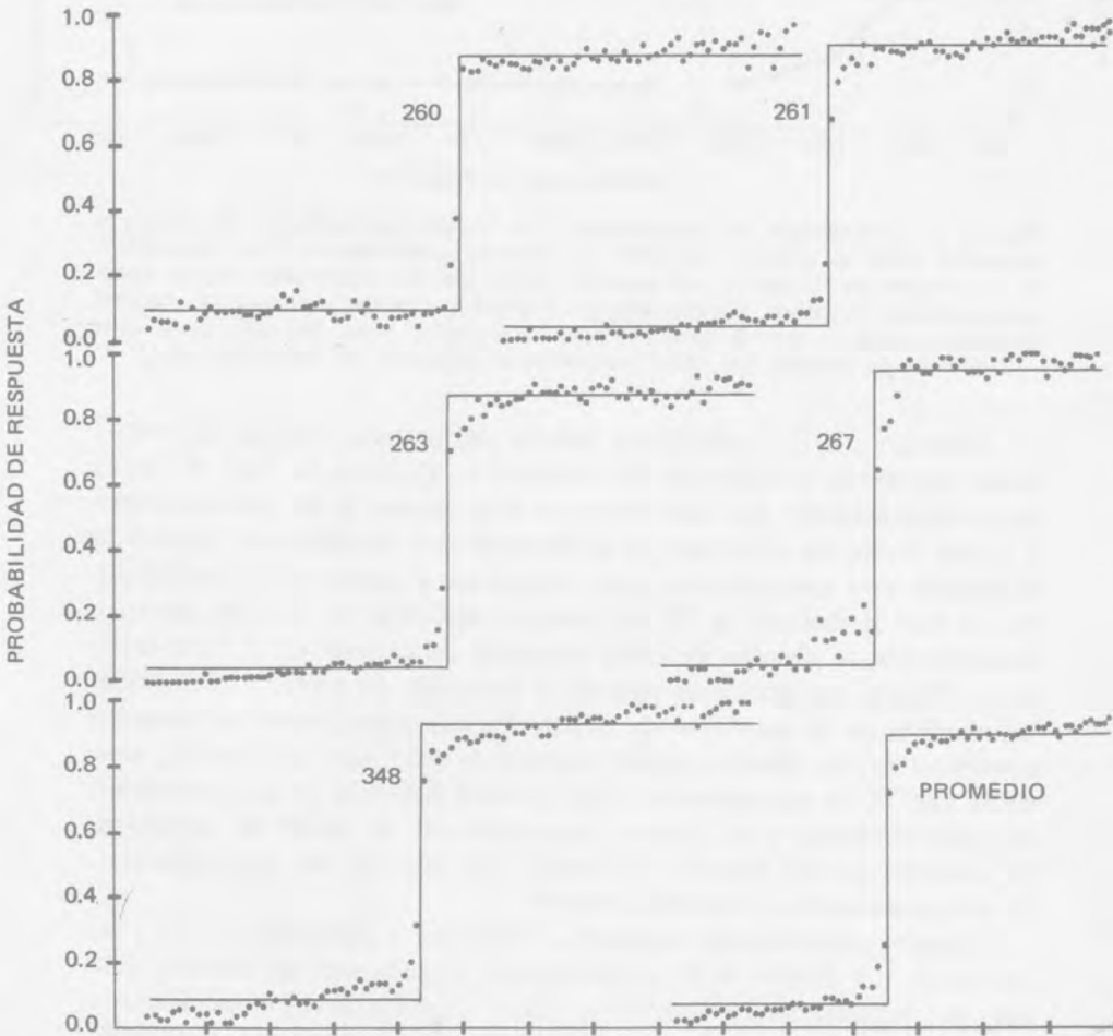
Figura 7. Probabilidad de respuesta antes y después del punto de corte, para cinco pájaros en IF 252 seg de ensayos discretos. La figura denominada "promedio" indica la media de esos cinco pájaros. La función sólida de escalón representa la conducta de dos estados perfectos. Cada unidad a lo largo de la abscisa corresponde a 40 segundos (diez ensayos). Cada punto representa un ensayo. (Tomado de Schneider y Neuringer, Journal of the Experimental Analysis of Behavior , vol. 18, núm. 2, 1972, págs. 187-199. Copyright 1972 por la Society for the Experimental Analysis of Behavior, Inc.)
