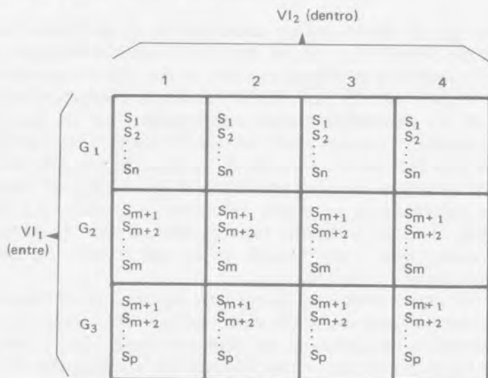
Figura 32. Esquema de un diseño 1 entre —1 dentro con tres valores de la VI_1 "entre" (tres grupos diferentes de sujetos) y cuatro valores de la VI_2 "dentro" (cada sujeto en cada uno de los tres grupos recibe los cuatro valores de la VI_2 ).
