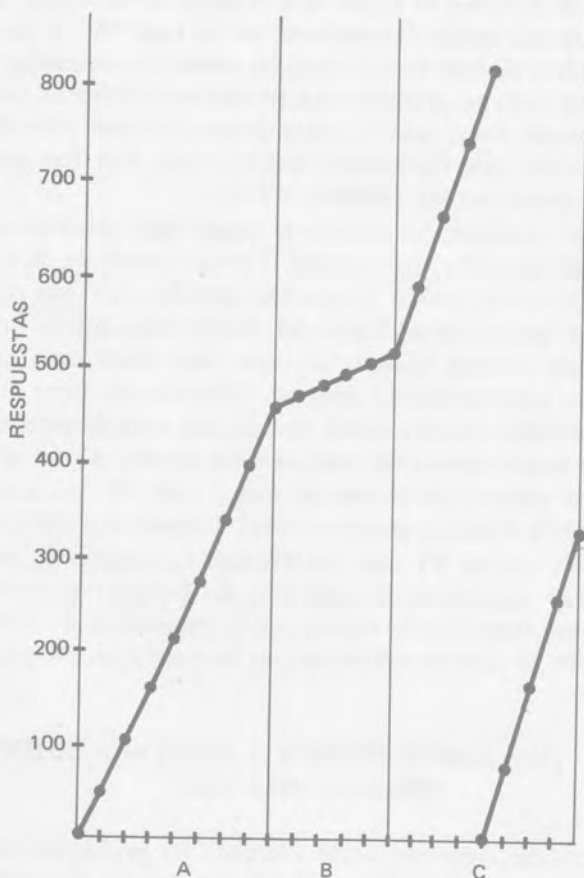
Figura 5. Registro acumulativo que muestra la tasa de una respuesta regida por una regla (fase B), comparada con la de línea base (A) y la recuperación opcional (C). (Tomado y adaptado de Moller, 1973.)
