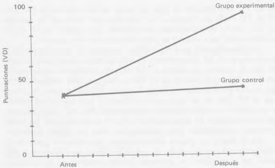
Figura 4. Datos ficticios que muestran un claro efecto de la VI sobre la VD.
