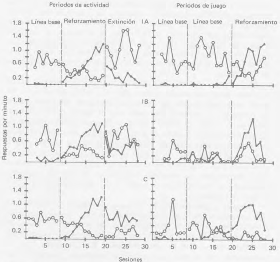
Figura 17. Número de sonidos emitidos, correctos e incorrectos, por minuto para todos los sujetos en el experimento 1. Cada punto representa las tasas totales correctas para todos los periodos de actividad o juego en cada sesión diaria. Los puntos sólidos indican los sonidos correctos, y los puntos en blanco representan los sonidos incorrectos. IA, IB e IC son tres diferentes sujetos. (Tomado y adaptado de Johnston y Johnston, Journal of Applied Behavior Analysis , vol. 5, núm. 3, otoño de 1972, págs. 233-246. Copyright por la Society for the Experimental Analysis of Behavior, Inc.)
