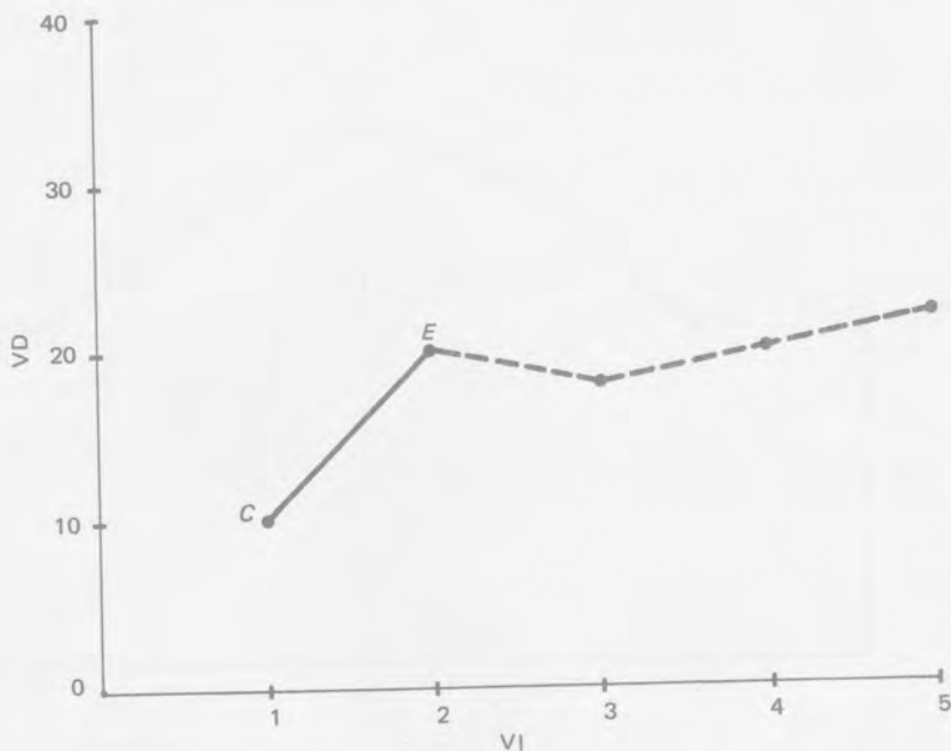
Figura 13. Datos ficticios que muestran una relación lineal directa entre la VI y la VD en el rango limitado a dos condiciones experimentales (línea continua) correspondientes a un diseño de dos grupos aleatorios . Esta relación no se sostiene en el resto del rango de la VI (línea punteada).
