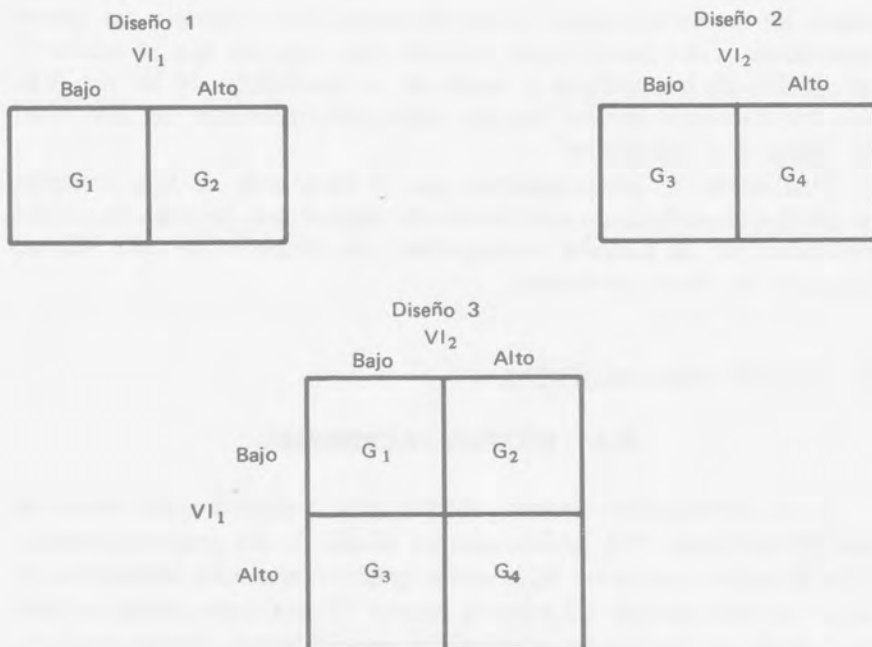
Figura 25. En la parte superior se muestra un esquema con dos diseños de dos grupos aleatorios separados. Cada VI asume dos valores y cada grupo asume sólo un valor de una VI. En la parte inferior se muestra un diseño factorial con dos VI, que asumen dos valores cada una, y cada grupo recibe un valor de cada VI.
