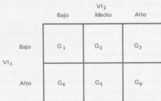
Figura 26. Un diseño factorial de 2 \times 3 . La primera VI tiene dos valores, la segunda tres y se forman seis grupos.
