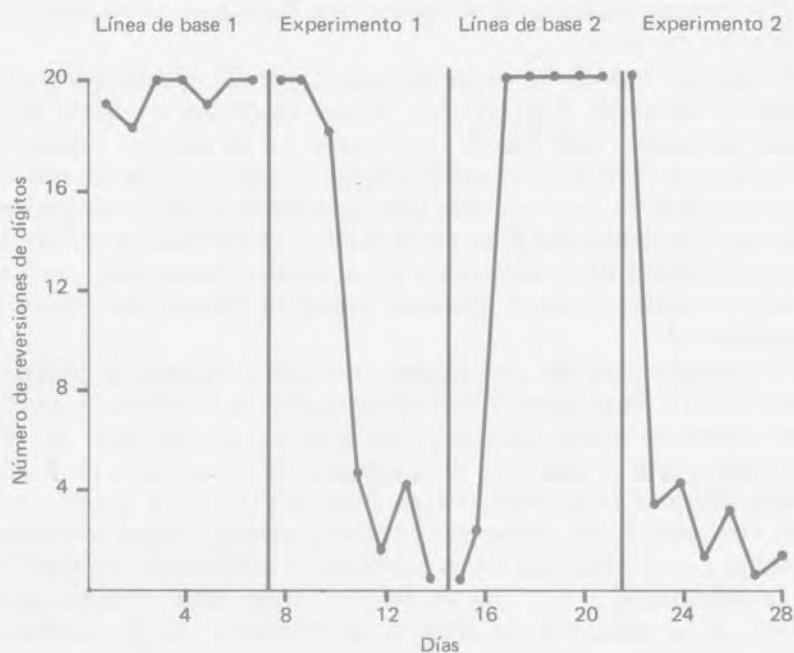
Figura 20. Número de reversiones de dígitos por día bajo condiciones de línea base y experimentales. Diseño A-B-A-B. (Tomado y adaptado de Hasazi y Hasazi, Journal of Applied Behavior Analysis , vol. 5, núm. 2, verano de 1972, págs. 157-162. Copyright 1972 por la Society for the Experimental Analysis of Behavior, Inc.)
