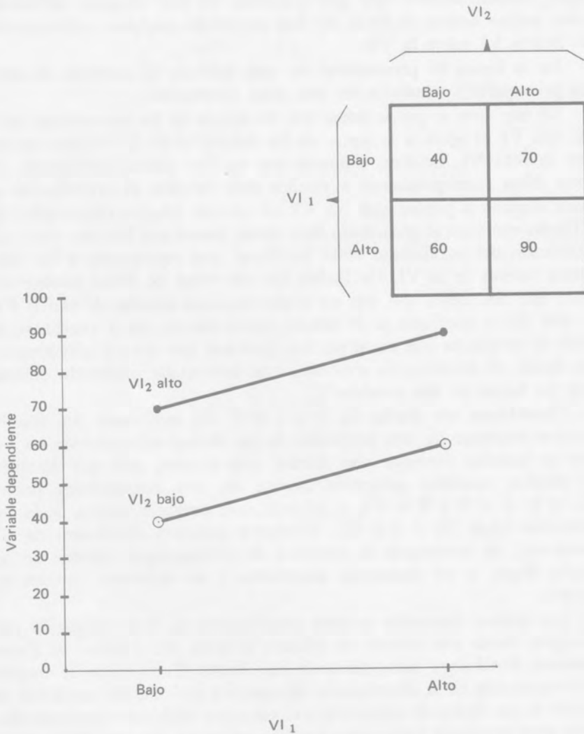
Figura 29. Datos ficticios y gráfica de un diseño factorial de 2 \times 2 que muestran un efecto principal.
