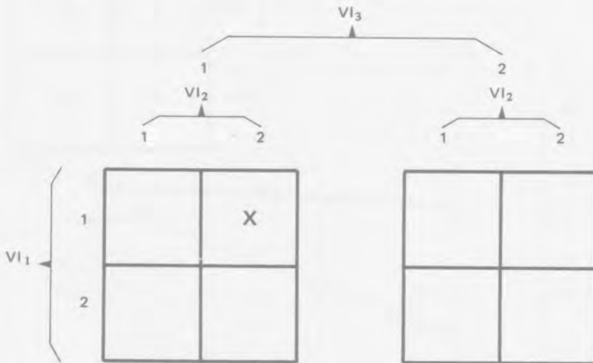
Figura 27. Un diseño factorial 2 \times 2 \times 2 . La celdilla marcada con una X corresponde a un grupo de sujetos que recibiría el valor 1 de la VI_1 , el valor 2 de la VI_2 y el valor 1 de la VI_3 .
