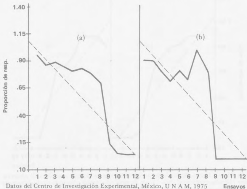
Figura 41 (a). Curva de posición serial obtenida con la serie completa de observaciones (40 observaciones) (b). Curva de posición serial obtenida exclusivamente con el bloque de observaciones más estables (10 observaciones).
