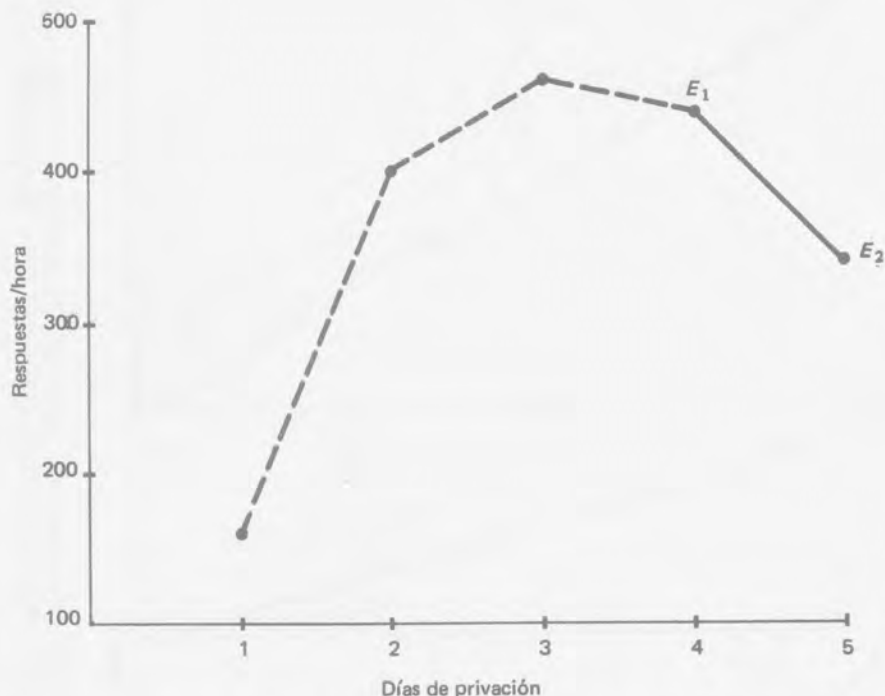
Figura 15. Datos ficticios que muestran una aparente relación inversa entre la VI (días de privación) y la VD (tasa de respuesta), sugerida por el uso de un diseño de dos grupos aleatorios (línea continua).
