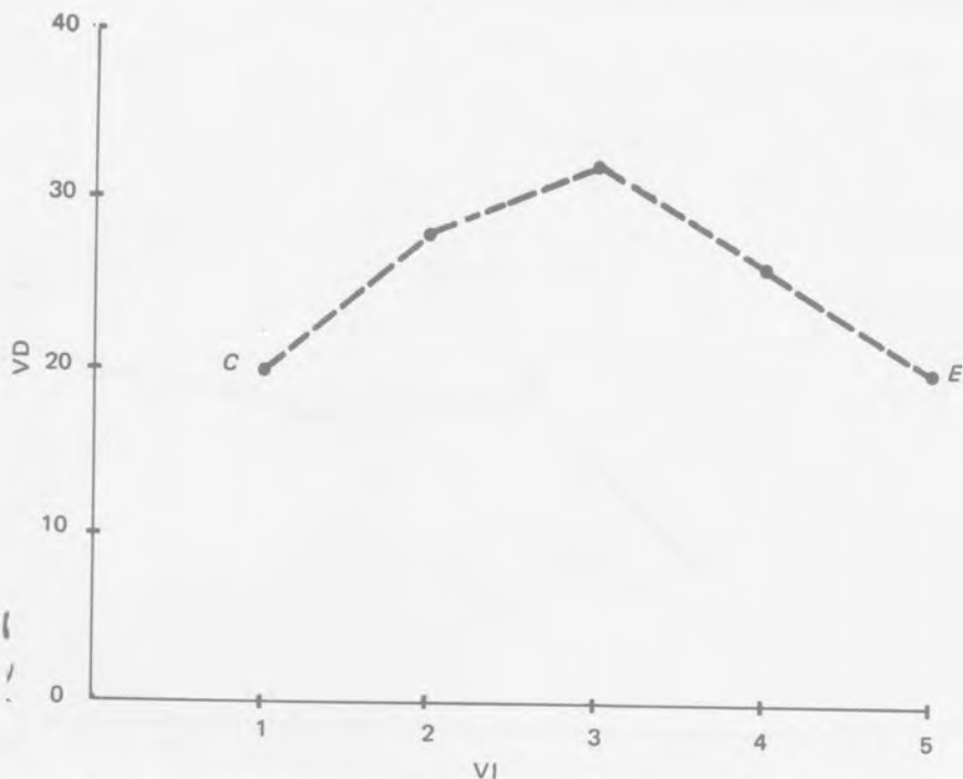
Figura 14. Datos ficticios que muestran una ausencia aparente del efecto de la VI sobre la VD. Nótese que no hay diferencia entre los valores de la VD en los puntos C y E.
