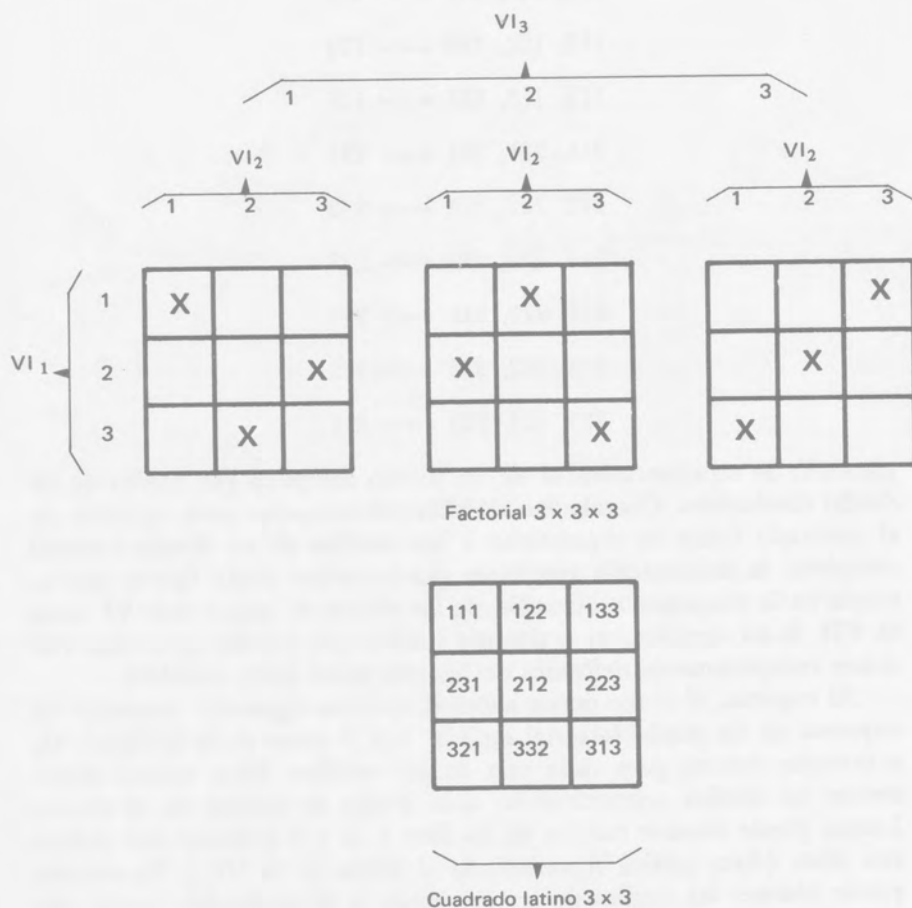
Figura 34. Celdillas de un diseño factorial de 3 \times 3 \times 3 (arriba) que se utilizaron para formar un cuadrado latino de 3 \times 3 . Los números en las celdillas del cuadrado latino indican las combinaciones de los valores de las tres VI.
