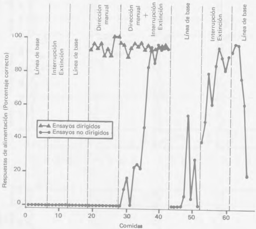
Figura 24. Porcentaje de respuestas de alimentación completadas correctamente por una niña de 6 años retardada profunda. Se le dieron cinco comidas ligeras durante un periodo de 6 horas cada día. Durante el procedimiento de "interrupción-extinción" la maestra impedía que la niña comiera, quitándole la comida de la mano durante una respuesta incorrecta. Durante el procedimiento de dirección manual, la maestra ayudó a la niña en los ensayos dirigidos, por medio de la dirección manual del movimiento apropiado. Durante la línea de base no se usó interrupción-extinción ni dirección manual. (Tomado y adaptado de O'Brien y Azrin, Journal of Applied Behavior Analysis , vol. 5, núm. 4, 1972, págs. 389-399. Copyright 1972 por la Society for the Experimental Analysis of Behavior, Inc.)
