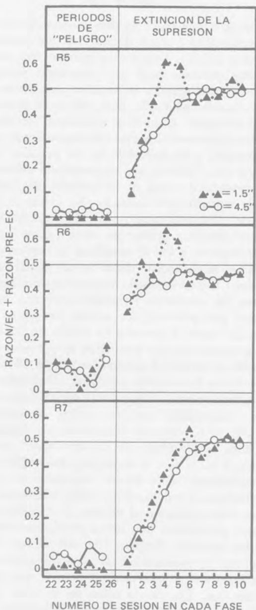
Figura 8. Razones de supresión para las cinco últimas sesiones de periodos de peligro de presentación de choque y para las subsecuentes diez sesiones de extinción. Los triángulos sólidos representan datos basados en las respuestas asociadas con una duración del reforzador de 1.5 segundos. Los círculos abiertos representan datos basados en respuestas a la palanca, asociados con una duración del reforzador de 4.5 segundos. (Tomado de De Villiers y Millenson, Journal of the Experimental Analysis of Behavior , vol. 18, núm. 2, 1972, págs. 287-294. Copyright 1972 por la Society for the Experimental Analysis of Behavior, Inc.)
