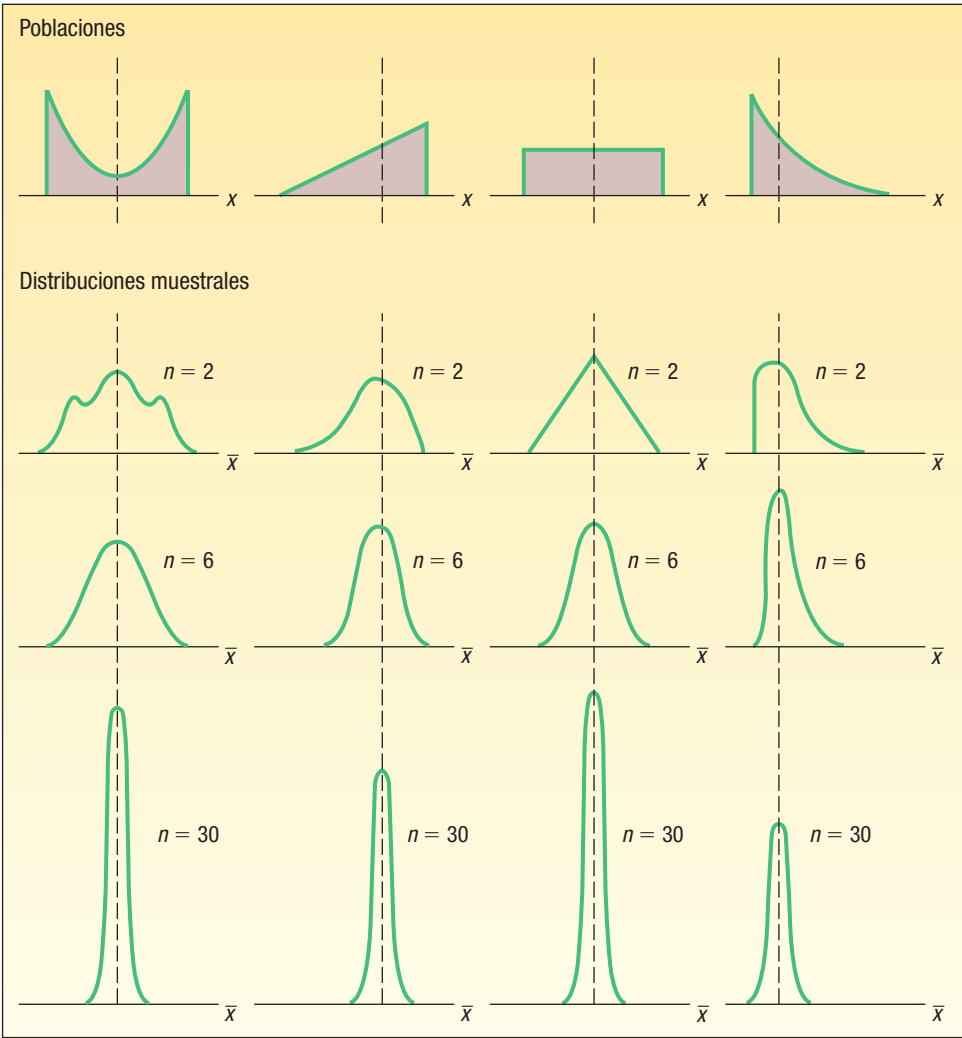
GRÁFICA 8-2 Resultados del teorema central del límite para diversas poblaciones
