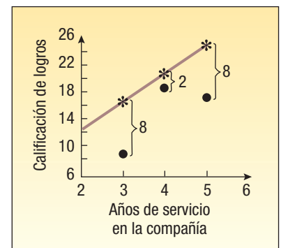
GRÁFICA 13-11 Recta diferente trazada con una regla
