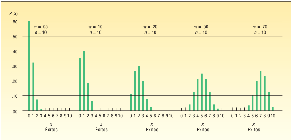
GRÁFICA 6-2 Representación gráfica de la distribución de probabilidad binomial para valores de \pi de 0.05, 0.10, 0.20, 0.50 y 0.70 con una n de 10
