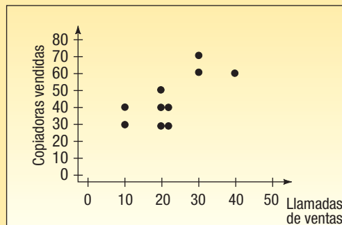
GRÁFICA 13-1 Diagrama de dispersión que representa las llamadas de ventas y las copiadoras vendidas
