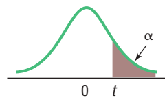
Prueba de cola derecha
