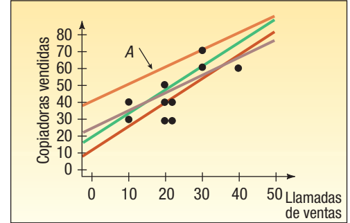
GRÁFICA 13-8 Cuatro rectas superpuestas en el diagrama de dispersión
