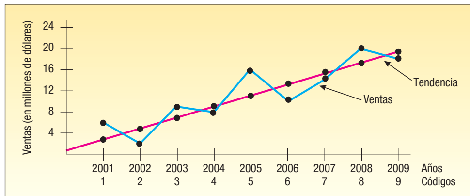
GRÁFICA 16-5 Recta ajustada a los datos de ventas
