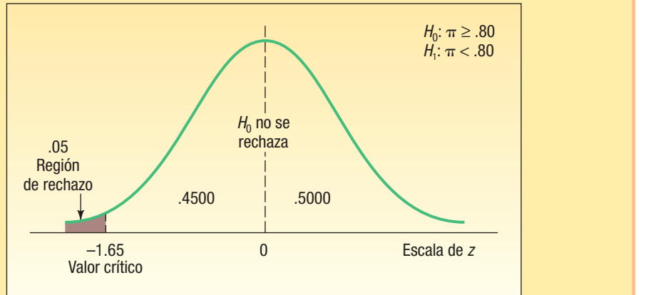
GRÁFICA 10-8 Región de rechazo del nivel de significancia de 0.05, prueba de una cola
