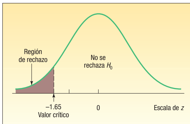
GRÁFICA 10-2 Distribución muestral del estadístico z , prueba de cola izquierda, nivel de significancia de 0.05
