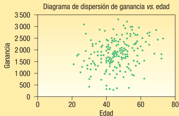
GRÁFICA 13-5 Diagrama de dispersión de los datos de Applewood Auto Group
