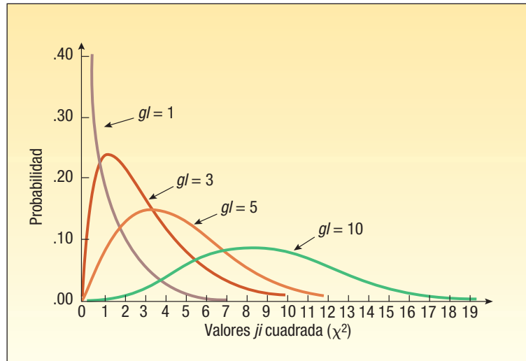
GRÁFICA 17-2 Distribuciones ji cuadrada de grados de libertad seleccionados
