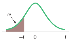
Prueba de cola izquierda
