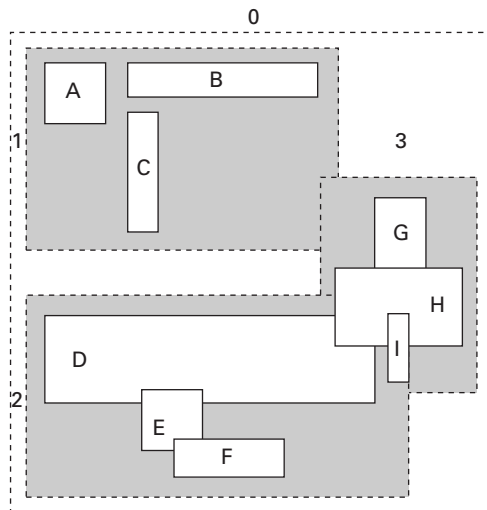
FIGURA 23.6. Árbol R.
